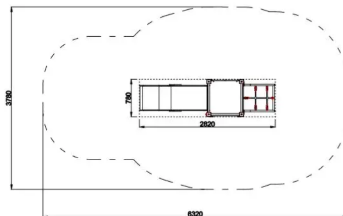
Rys. 1. Wymiary urządzenia i strefy bezpieczeństwa
