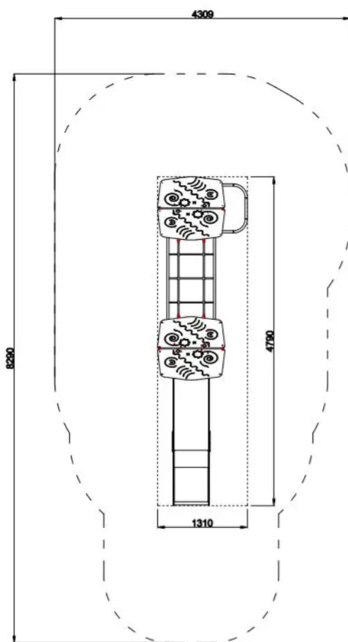
Rys. 1. Wymiary urządzenia i strefy bezpieczeństwa
