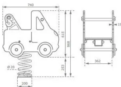
Rys. 1. Wymiary urządzenia
