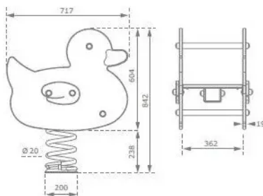
Rys. 1. Wymiary urządzenia
