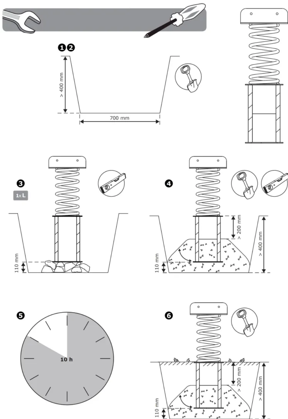
Rys. 2. Montaż
