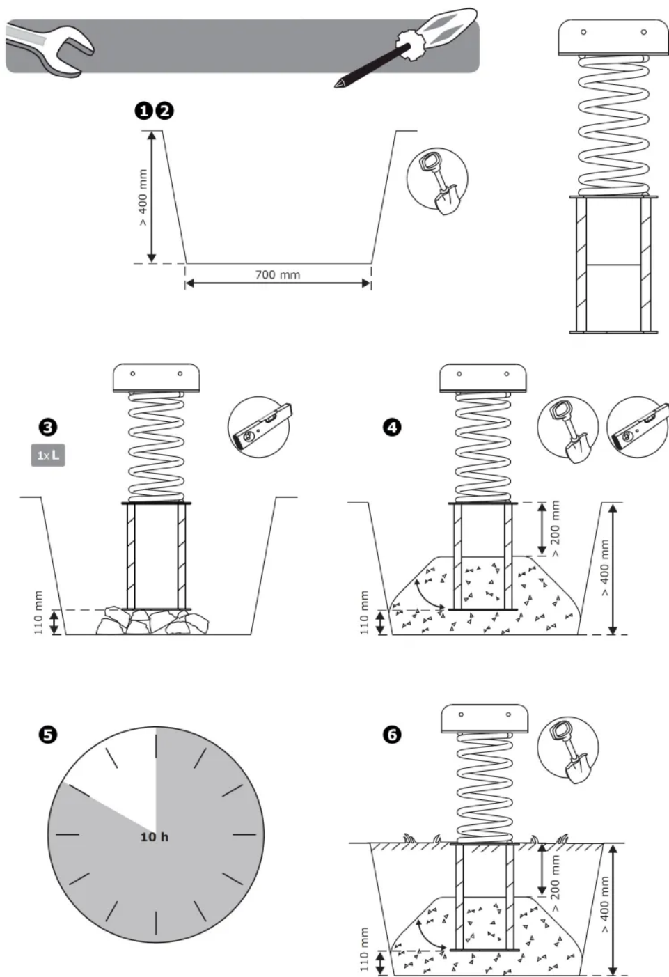
Rys. 2. Montaż
