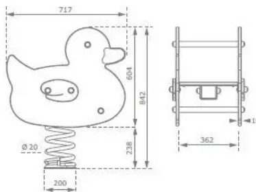
Rys. 1. Wymiary urządzenia
