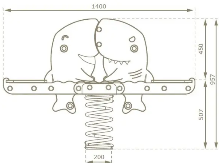
Rys. 1. Wymiary urządzenia
