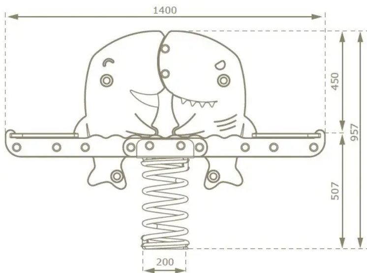
Rys. 1. Wymiary urządzenia
