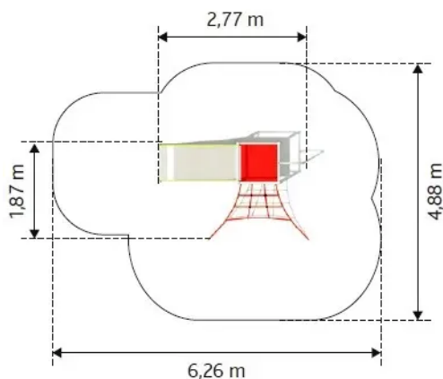
Rys. 1. Wymiary urządzenia i strefy bezpieczeństwa
