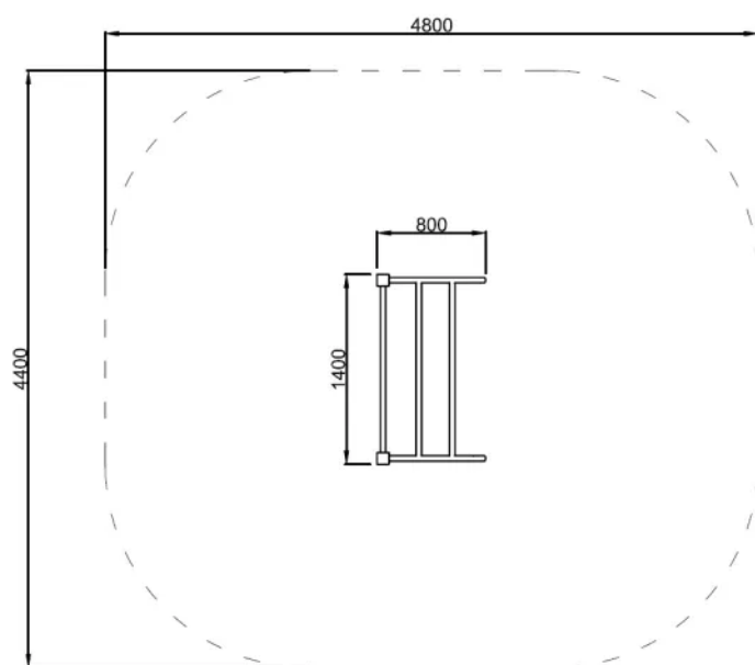
Rys. 1. Wymiary urządzenia i strefy bezpieczeństwa
