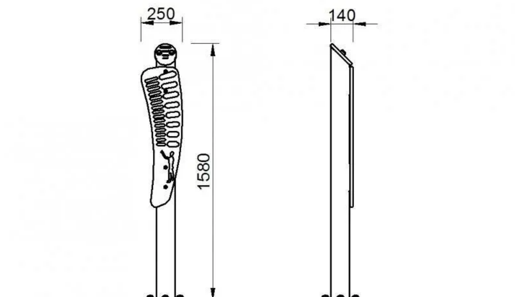
Rys. 1. Wymiary urządzenia
