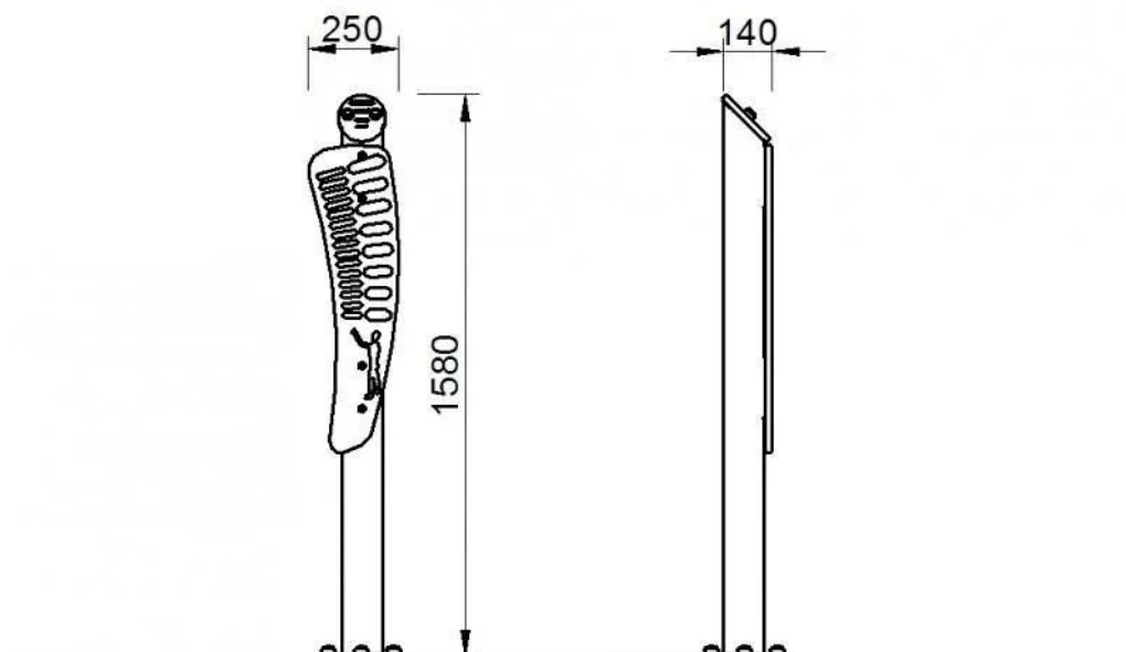
Rys. 1. Wymiary urządzenia
