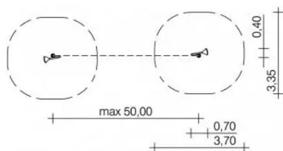
Rys. 1. Wymiary urządzenia i strefy bezpieczeństwa
