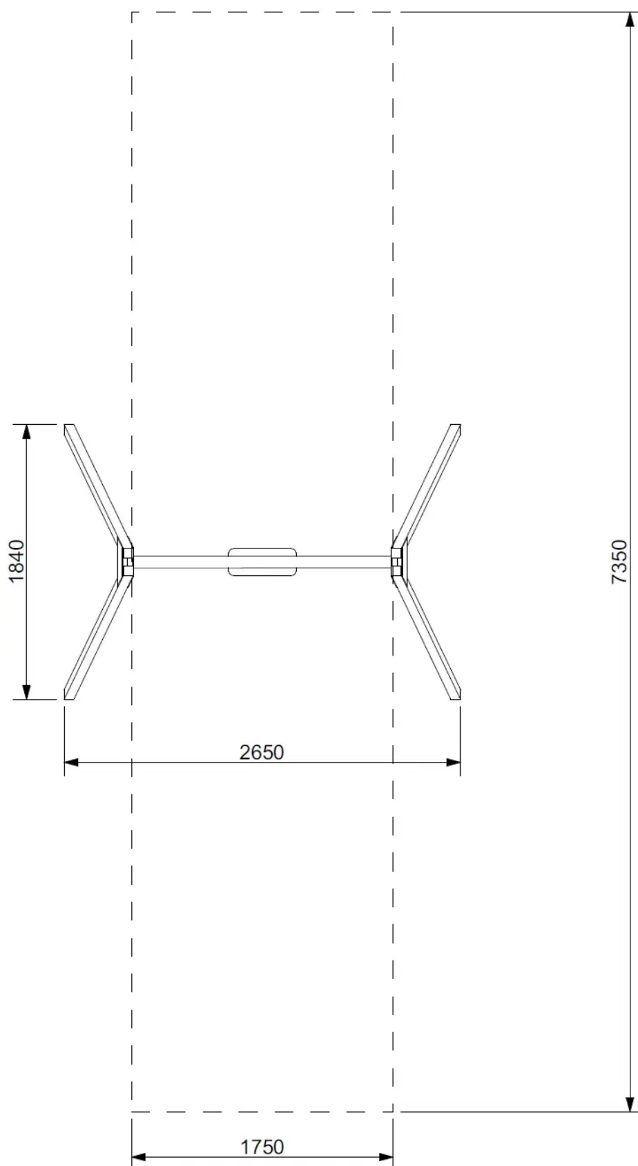
Rys. 1. Wymiary urządzenia i strefy bezpieczeństwa
