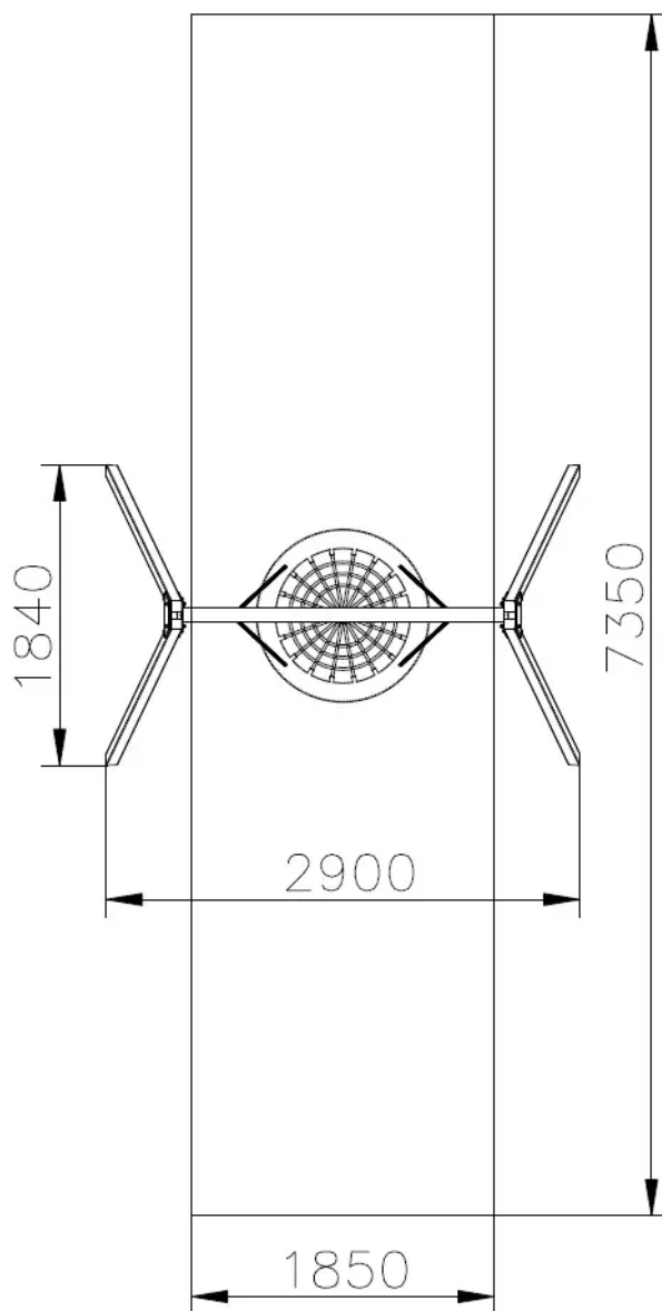
Rys. 1. Wymiary urządzenia i strefy bezpieczeństwa
