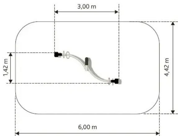
Rys. 1. Wymiary urządzenia i strefy bezpieczeństwa
