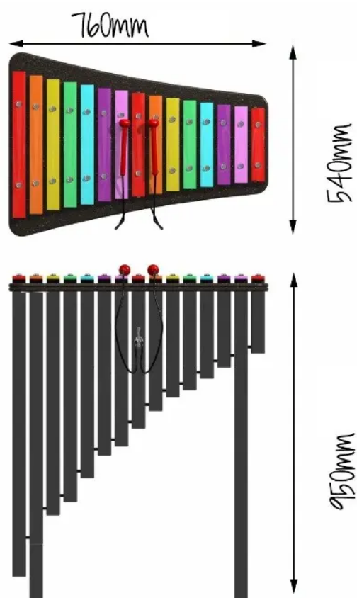
Rys. 1. Wymiary urządzenia
