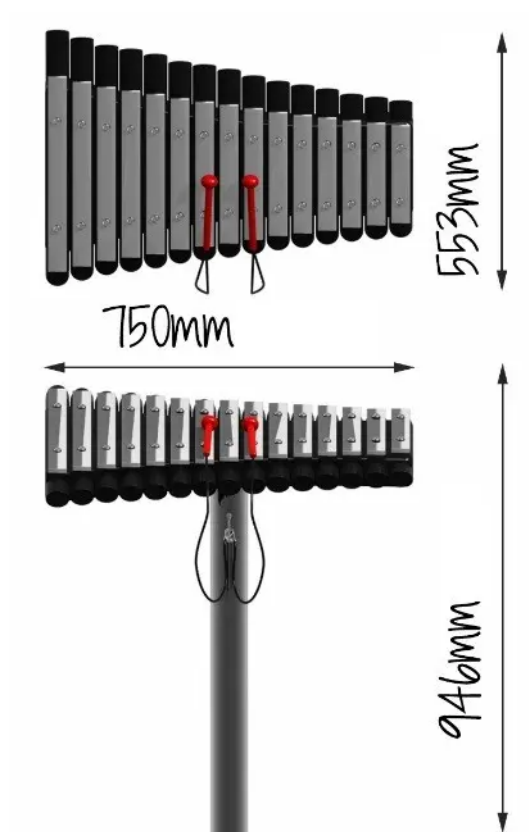
Rys. 1. Wymiary urządzenia
