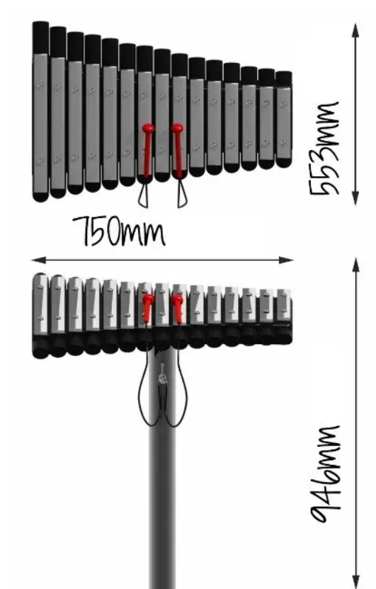
Rys. 1. Wymiary urządzenia
