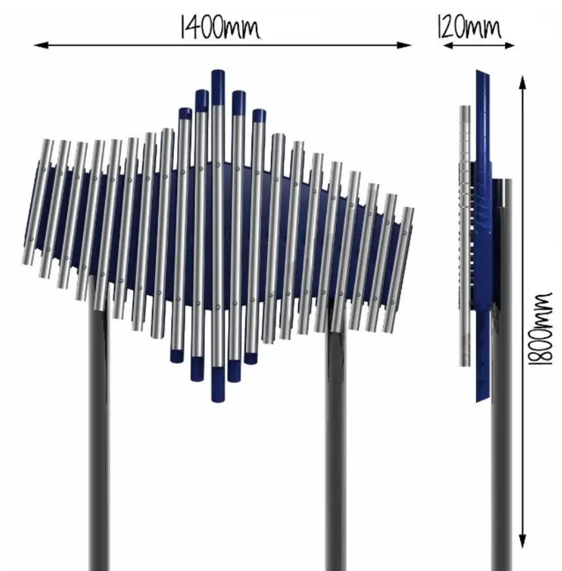
Rys. 1. Wymiary urządzenia
