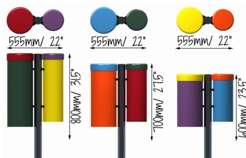
Rys. 1. Wymiary urządzenia
