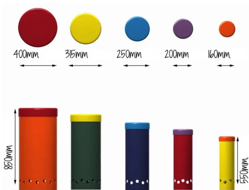
Rys. 1. Wymiary urządzenia
