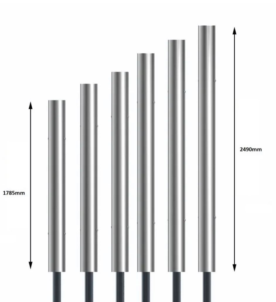
Rys. 1. Wymiary urządzenia
