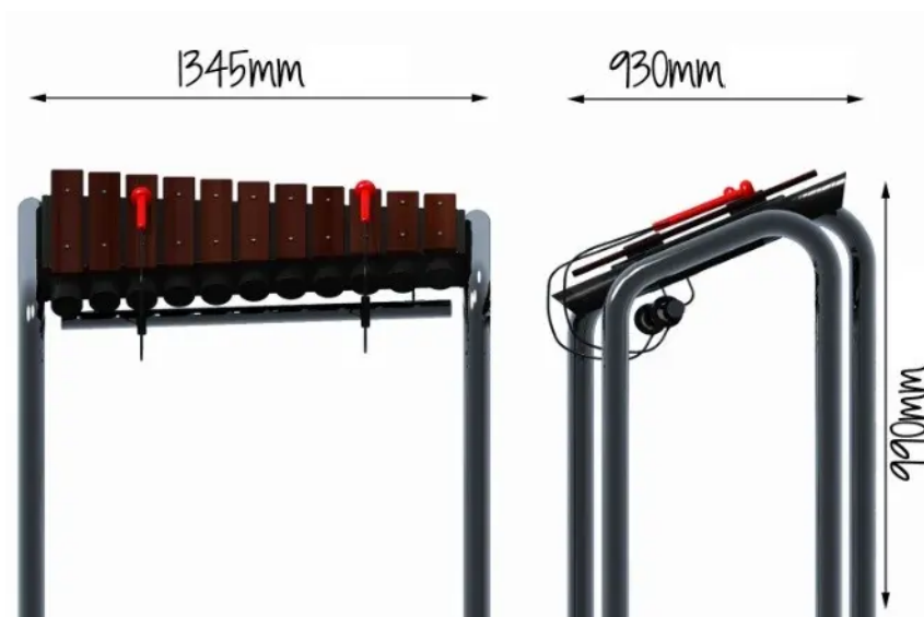
Rys. 1. Wymiary urządzenia
