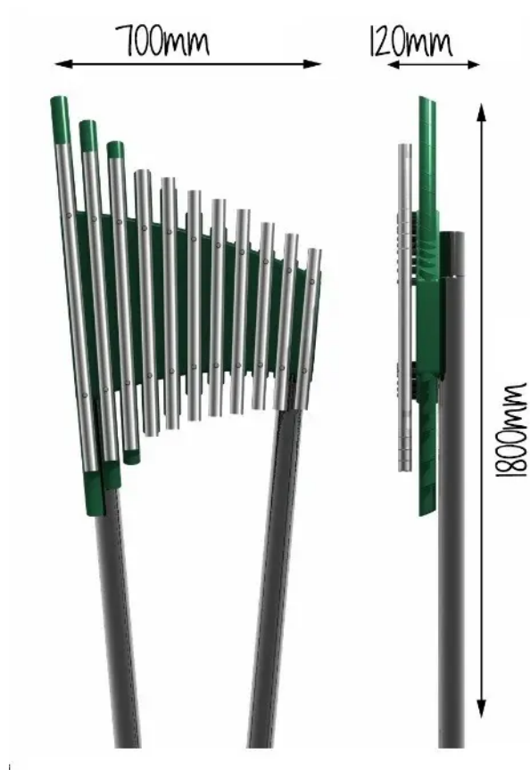
Rys. 1. Wymiary urządzenia
