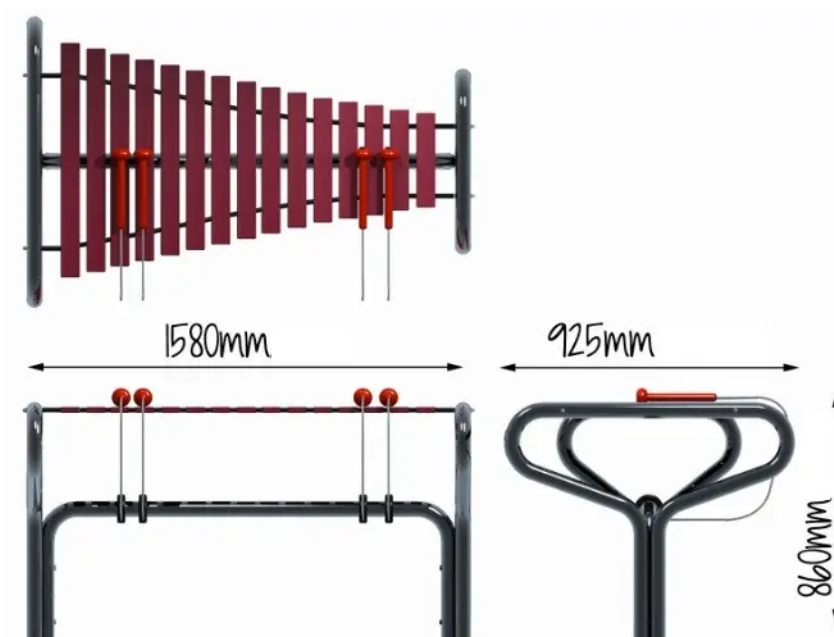
Rys. 1. Wymiary urządzenia
