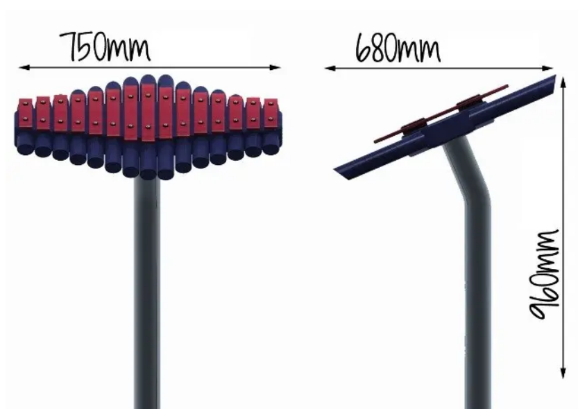
Rys. 1. Wymiary urządzenia
