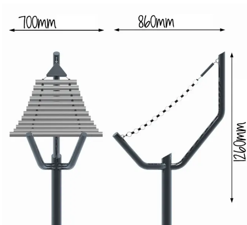
Rys. 1. Wymiary urządzenia
