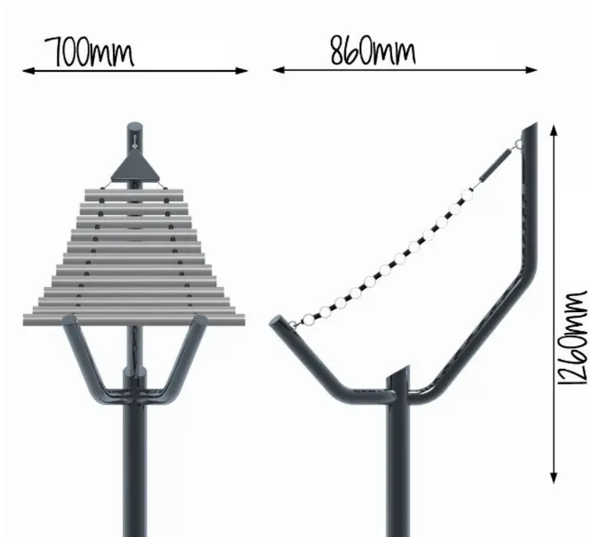
Rys. 1. Wymiary urządzenia
