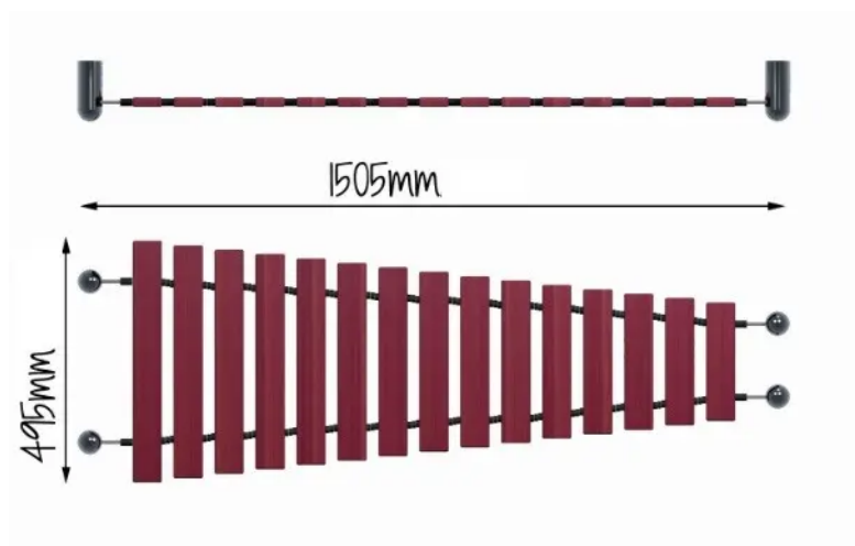
Rys. 1. Wymiary urządzenia
