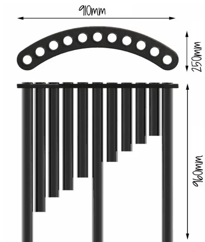
Rys. 1. Wymiary urządzenia
