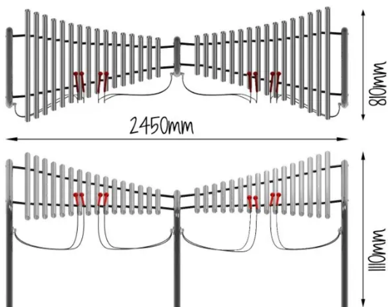
Rys. 1. Wymiary urządzenia
