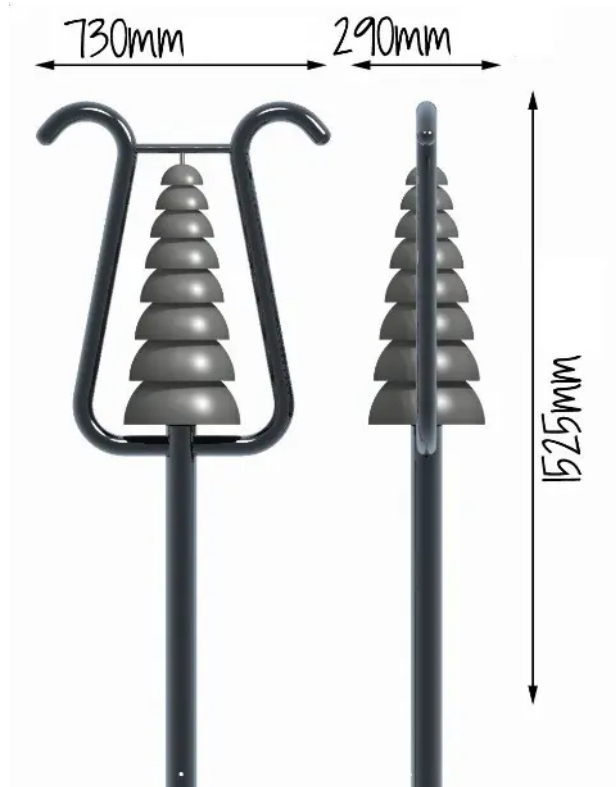
Rys. 1. Wymiary urządzenia
