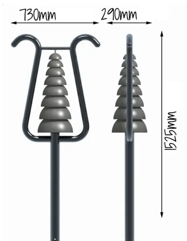
Rys. 1. Wymiary urządzenia
