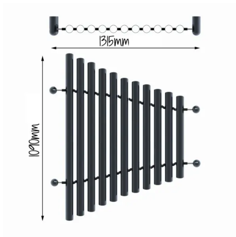
Rys. 1. Wymiary urządzenia
