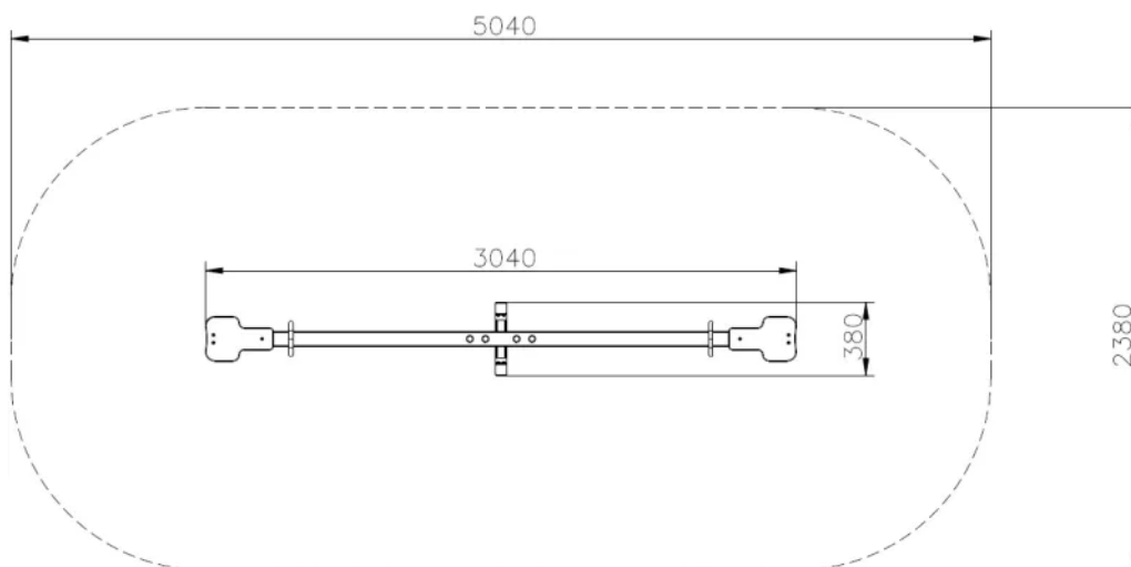
Rys. 1. Wymiary urządzenia i strefy bezpieczeństwa
