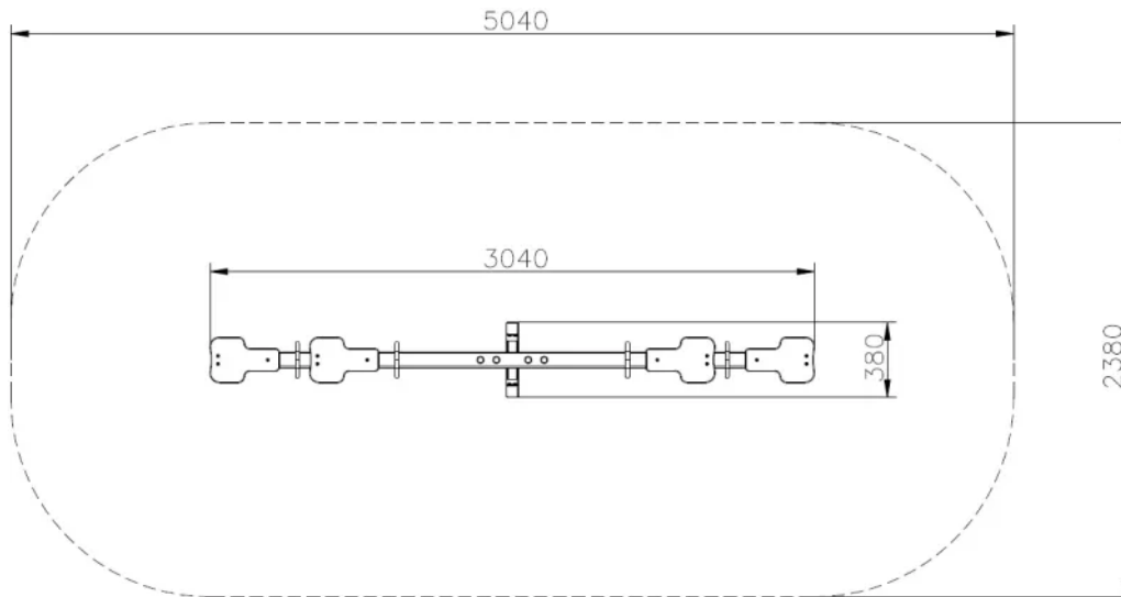
Rys. 1. Wymiary urządzenia i strefy bezpieczeństwa
