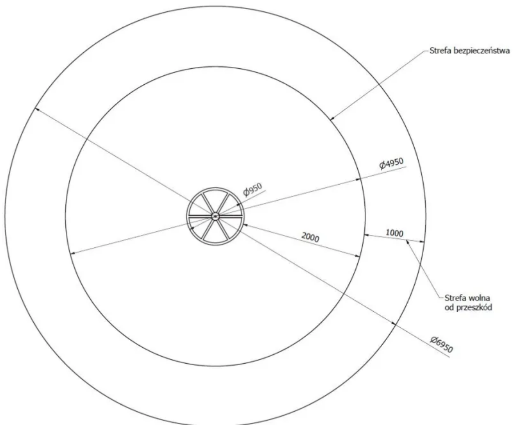
Rys. 2. Strefa wolna od przeszkód
