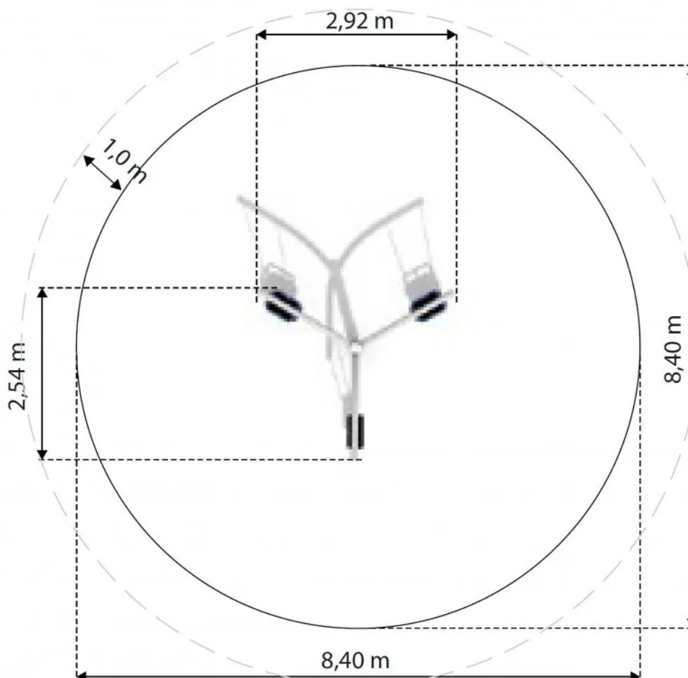
Zał.1. Wymiary urządzenia i strefy bezpieczeństwa
