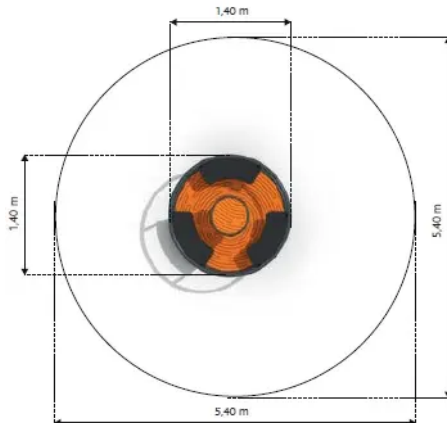
Rys. 1. Wymiary urządzenia i strefy bezpieczeństwa
