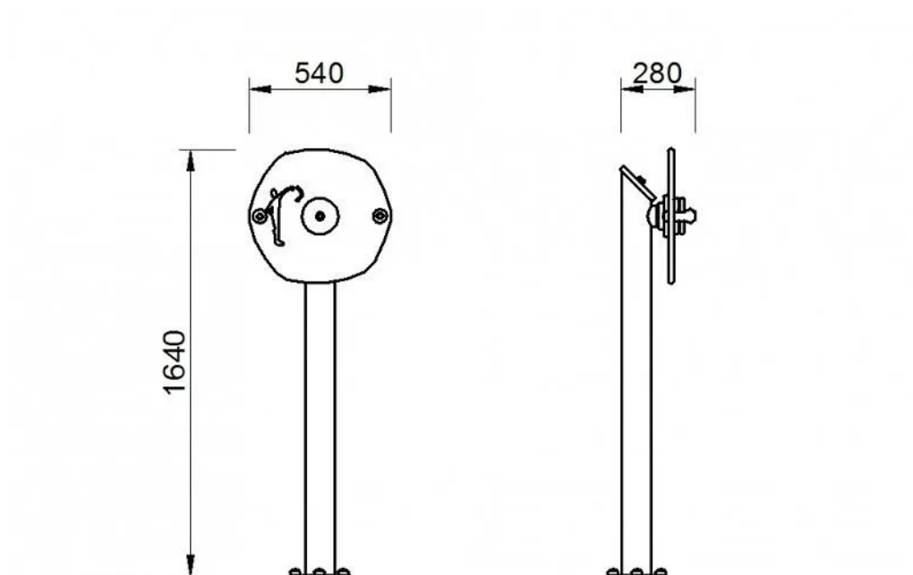
Rys. 1. Wymiary urządzenia
