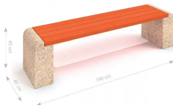
Rys. 1. Wymiary urządzenia
