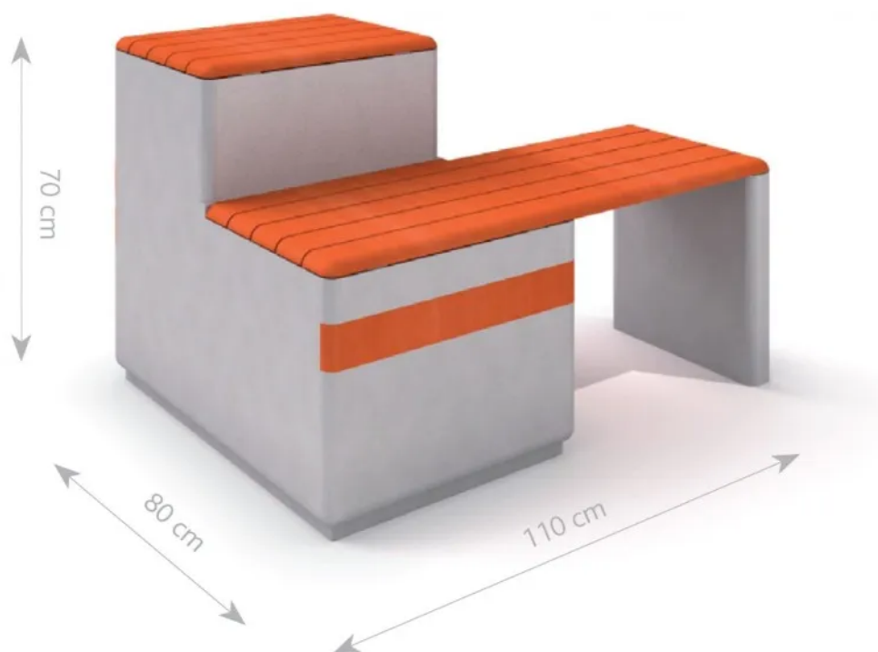
Rys. 1. Wymiary urządzenia
