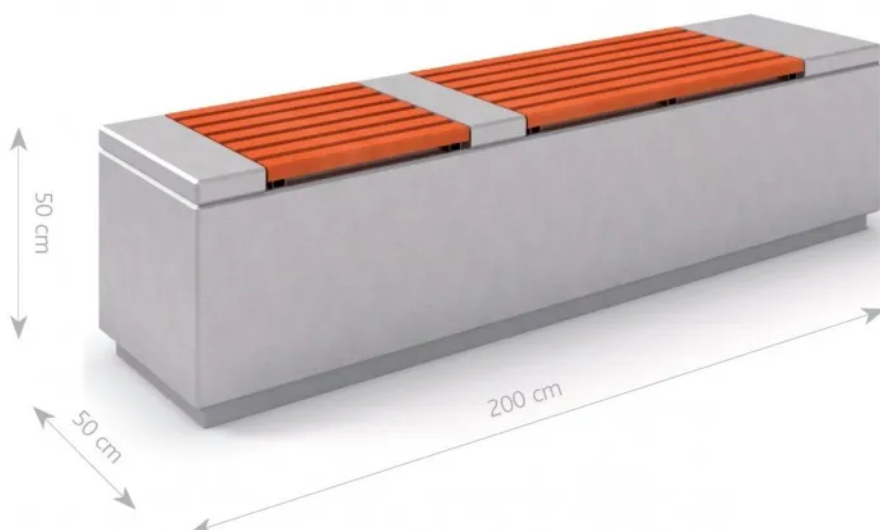
Rys. 1. Wymiary urządzenia
