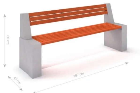
Rys. 1. Wymiary urządzenia
