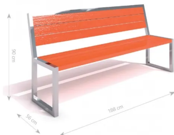
Rys. 1. Wymiary urządzenia
