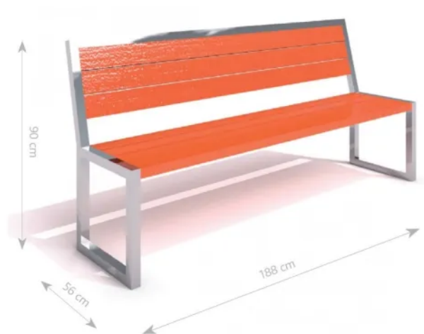
Rys. 1. Wymiary urządzenia
