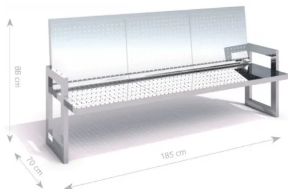
Rys. 1. Wymiary urządzenia
