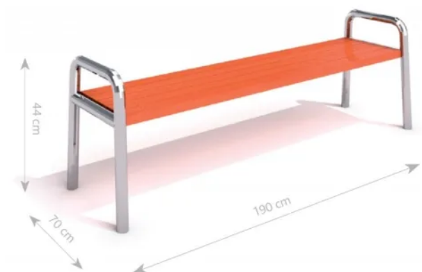
Rys. 1. Wymiary urządzenia
