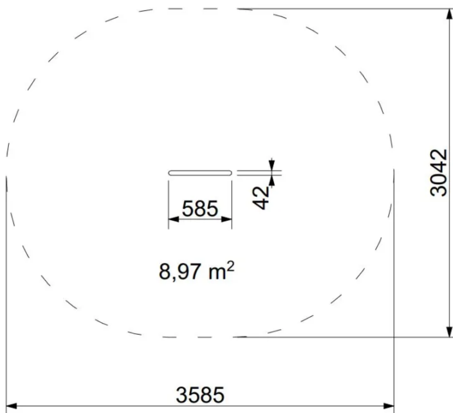
Rys. 1. Wymiary urządzenia
