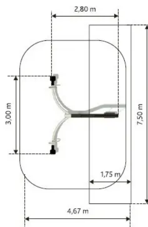
Rys. 1. Wymiary urządzenia i strefy bezpieczeństwa
